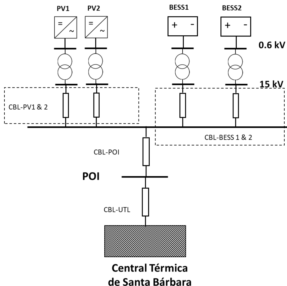
Figura 1. Esquema da rede elétrica da CSFH, ligada à rede de distribuição e transporte da ilha do Faial no Poi.
