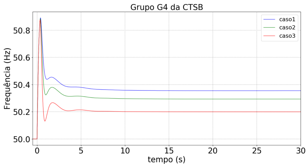
Figura 47. Velocidade do gerador síncrono para os diferentes casos – Cenário 3.
