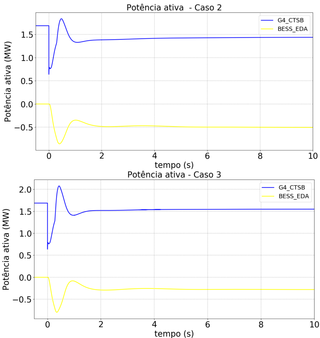
Figura 43. Resposta de potência ativa do gerador síncrono e BESS (em primeiro - caso1, em segundo - caso2 e em terceiro - caso3) – Cenário 1.
