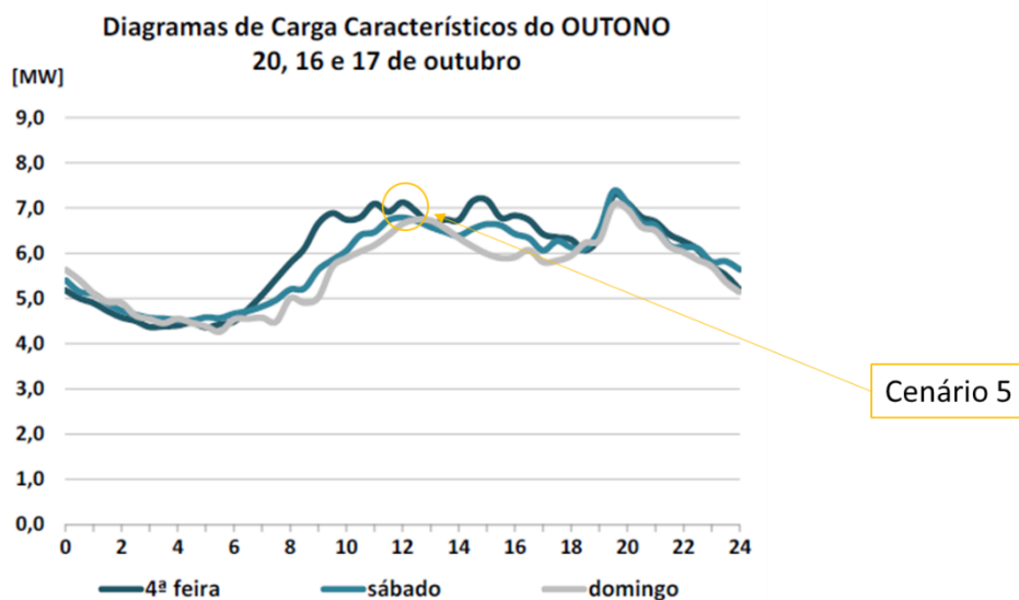
Figura 10. Diagramas de cargas típicas fornecidos pela EDA e pontos do diagrama escolhidos para a definição dos cenários (considerando um ligeiro aumento de carga).
