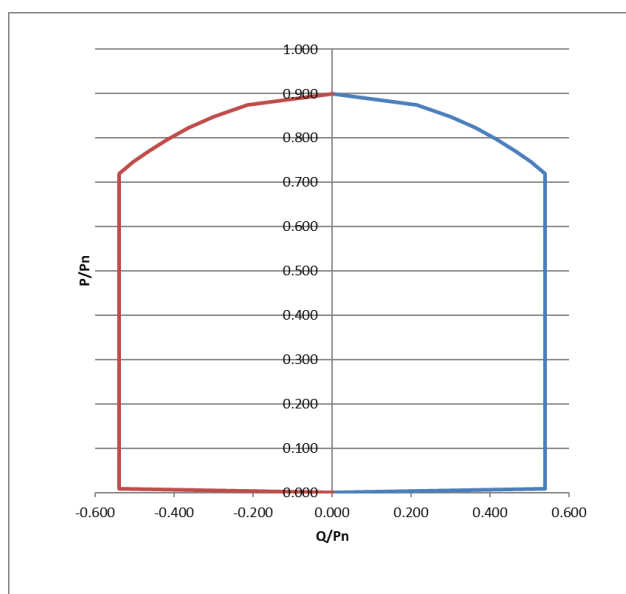
Figura 5. Curva característica P/Q dos conversores a instalar na CSFH.
