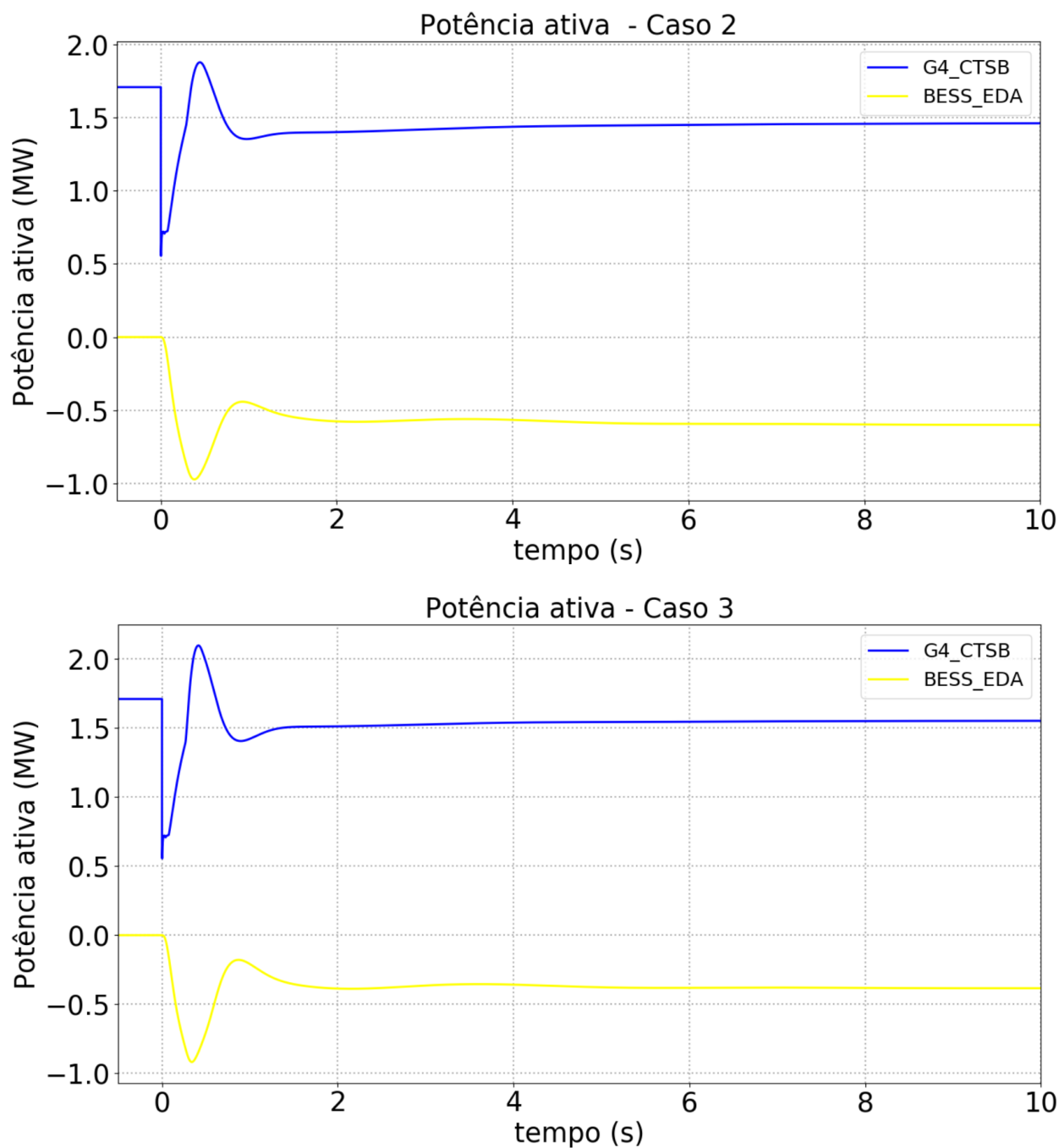
Figura 55. Resposta de potência ativa do gerador síncrono e BESS (em primeiro - caso1, em segundo - caso2 e em terceiro - caso3) – Cenário 5.
