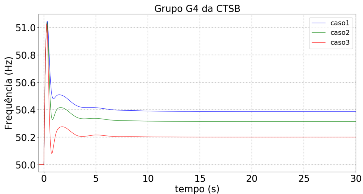
Figura 53. Velocidade do gerador síncrono para os diferentes casos – Cenário 5.
