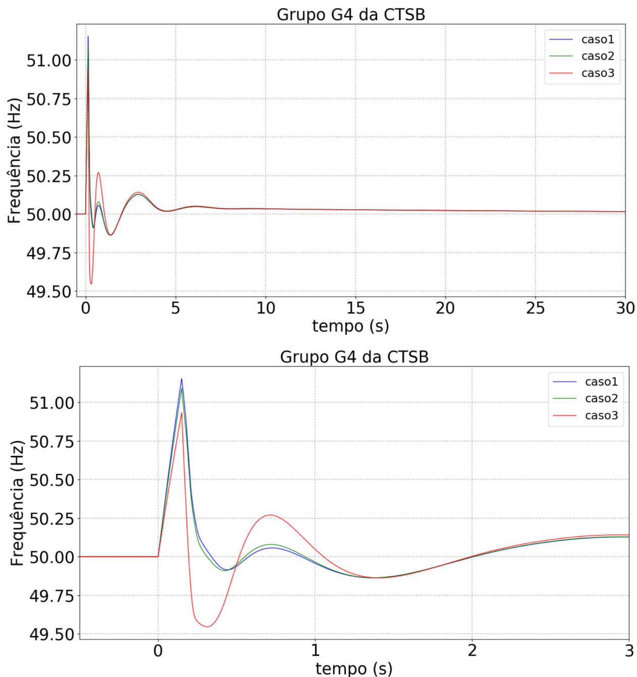
Figura 33. Velocidade do gerador síncrono (em cima – tempo total de simulação, em baixo – detalhe dos 0 a 3 s) – Cenário 4.
