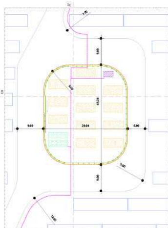
P2 - Substação 1 : 500
