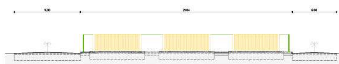
Substação - Corte BB' 1 : 200
