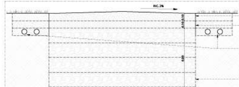
PORMENOR CONSTRUTIVO PERFIL DO ARRUIAMENTO EM GRAVILHA PARA ACESSO A VEÍCULOS PESADOS NO INTERIOR DO LOTE CORTE 1:20
