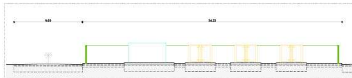
Substação - Corte AA' 1 : 200
