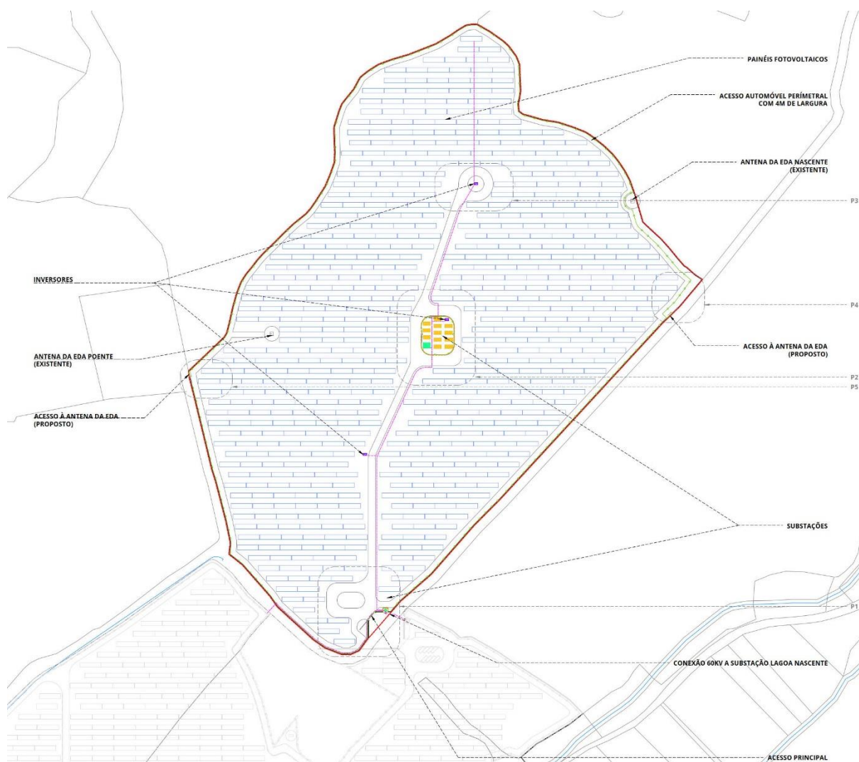
Figura 2.2 | Planta geral prevista do empreendimento (Elemento do Pedido de Informação Prévia, disponibilizado pelo promotor - © Millenniarch)
