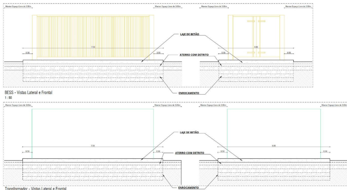
Figura 2.5 | Detalhes da BESS e transformador (Elemento do Pedido de Informação Prévia, disponibilizado pelo promotor - © Millenniarch)
