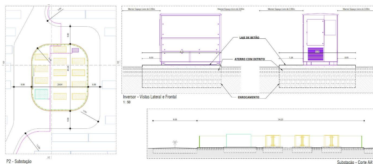
Figura 2.4 | Detalhes da subestação e do inversor (Elemento do Pedido de Informação Prévia, disponibilizado pelo promotor - © Millenniarch)
