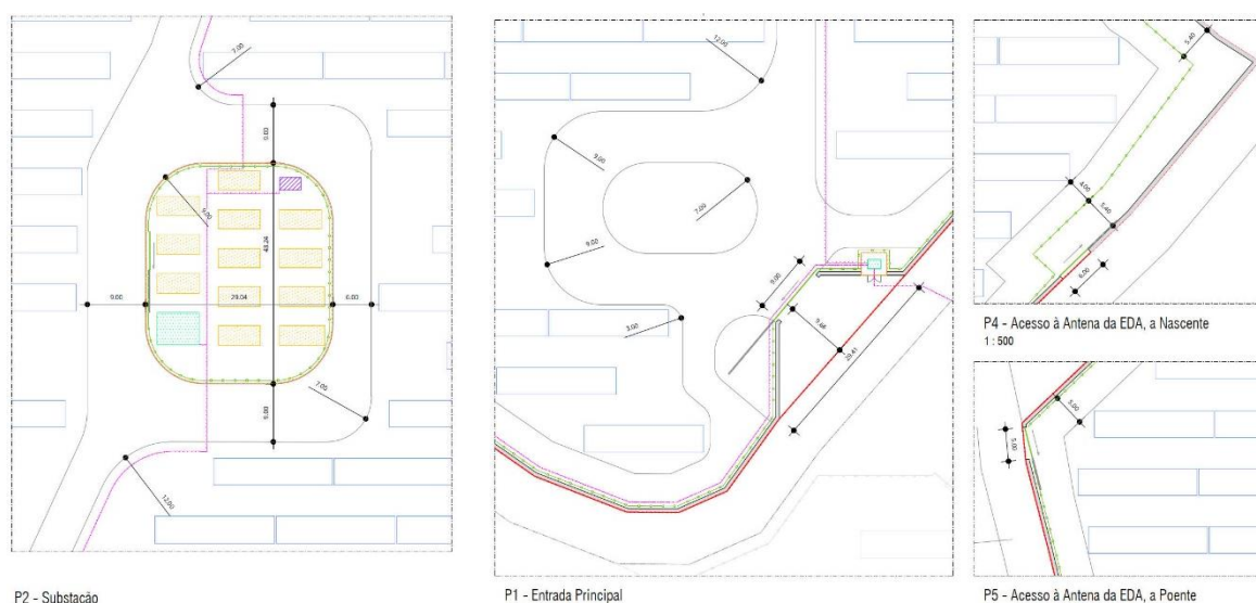
Figura 2.3 | Plantas Gerais dos Acessos, Arruamentos e Subestações (Elemento do Pedido de Informação Prévia, disponibilizado pelo promotor - © Millenniarch)
