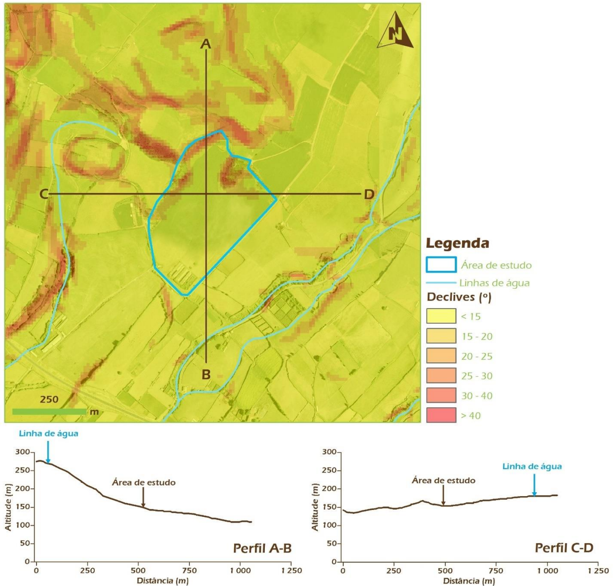
Figura 2.3 | Representação esquemática do mapa de declives da área de estudo e perfis topográficos interpretativos (base geográfica de https://ot.azores.gov.pt/Informacao-Geografica.aspx?ilha=saomiguel )
