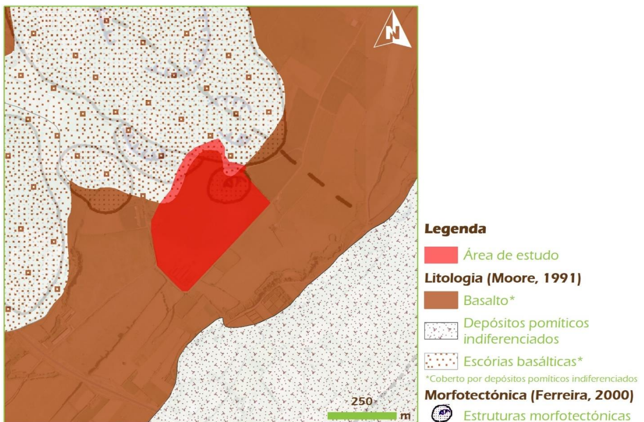
Figura 2.7 | Cartografia litológica da área de estudo e envolvente (adaptado de Moore, 1991; base geográfica de https://ot.azores.gov.pt/Informacao-Geografica.aspx?ilha=saomiguel )
